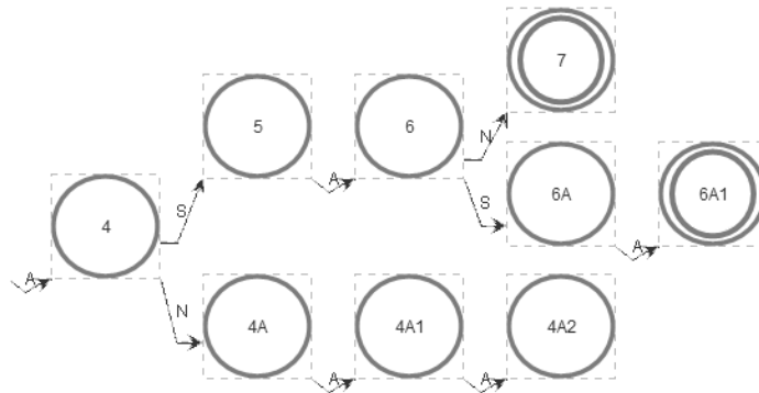
Fig. 7. Fragmento del grafo de estados en el simulador de autómatas finitos.
