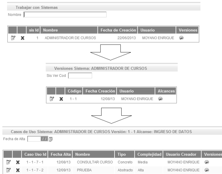
Fig. 2. Consulta de Casos de Uso de un Sistema.
